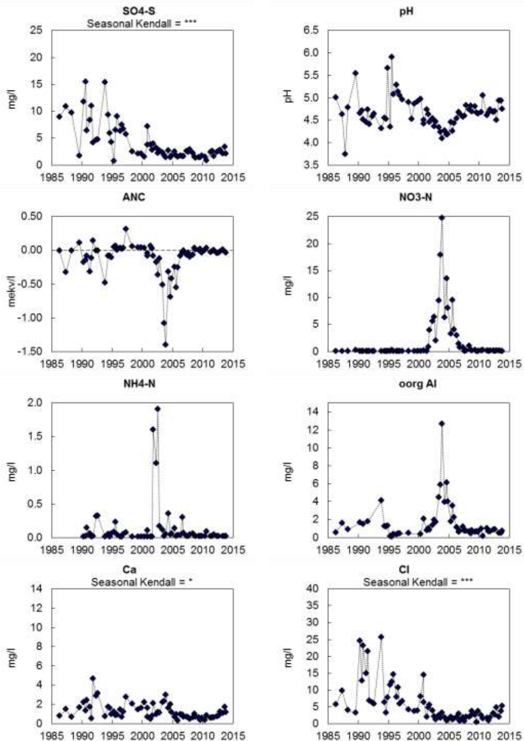
Figur B1:9. Markvattenkemi vid Kallgårdsmåla, K 10 . Sulfatsvavel (SO 4 -S); pH; markvattnets syraneutraliserande förmåga (ANC); nitratkväve (NO 3 -N), ammoniumkväve (NH 4 -N), oorganiskt aluminium (oorg Al); kalciumhalt (Ca 2+ ) samt klorid (Cl). Saknade värden innebär oftast att marken varit för torr. Trendanalys har genomförts med hjälp av Seasonal-Kendall metodik och signifikansnivåer anges, ovanför respektive diagram, i de fall där signifikanta trender påvisats.
