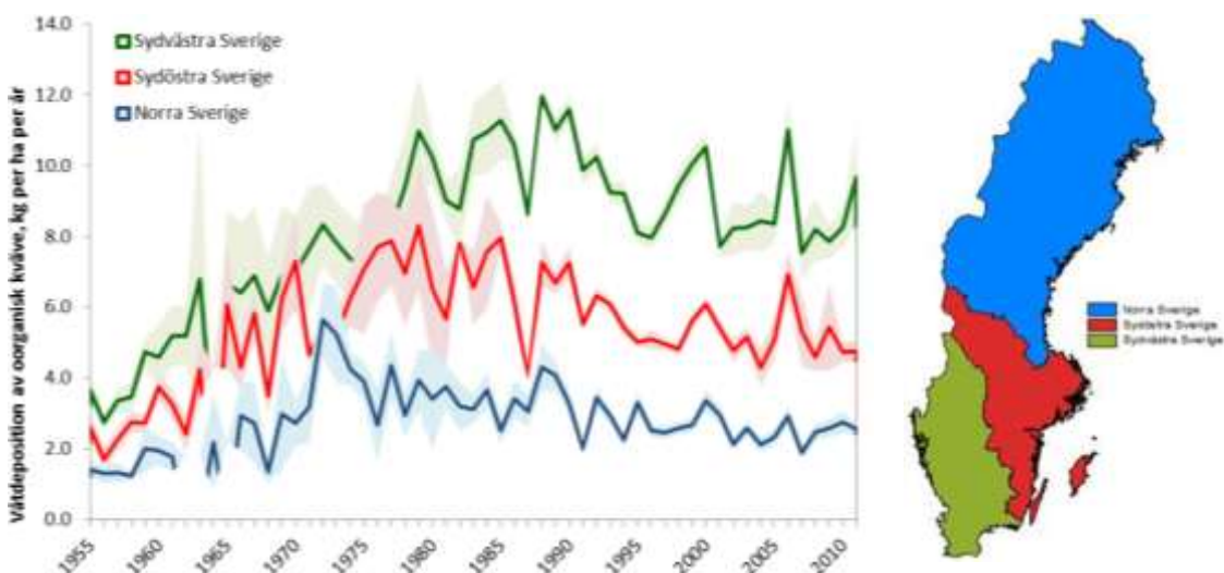
Figur 14. Nedfallet av oorganiskt kväve (NO 3 + NH 4 ) med våtdepositionen (kg/ha/år) i tre regioner (se karta) för åren 1955-2011. Utöver våtdepositionen finns ett litet inslag av torrdeposition från provtagningsutrustningen i provet. Linjerna visar årsvisa medelvärden från de lokaler som det finns mätdata från det aktuella året. Det färgade området kring linjerna visar medelfelet i data (Standard Error). Det är olika antal stationer olika år. Man ser att variationen i data minskade efter det att Krondroppsnetet startade 1985 främst på grund av att antalet mätstationer ökade. Efter 2003 har antalet mätplatser återigen minskat. Källa: IVL, 2013; Hansen m.fl., 2013.
