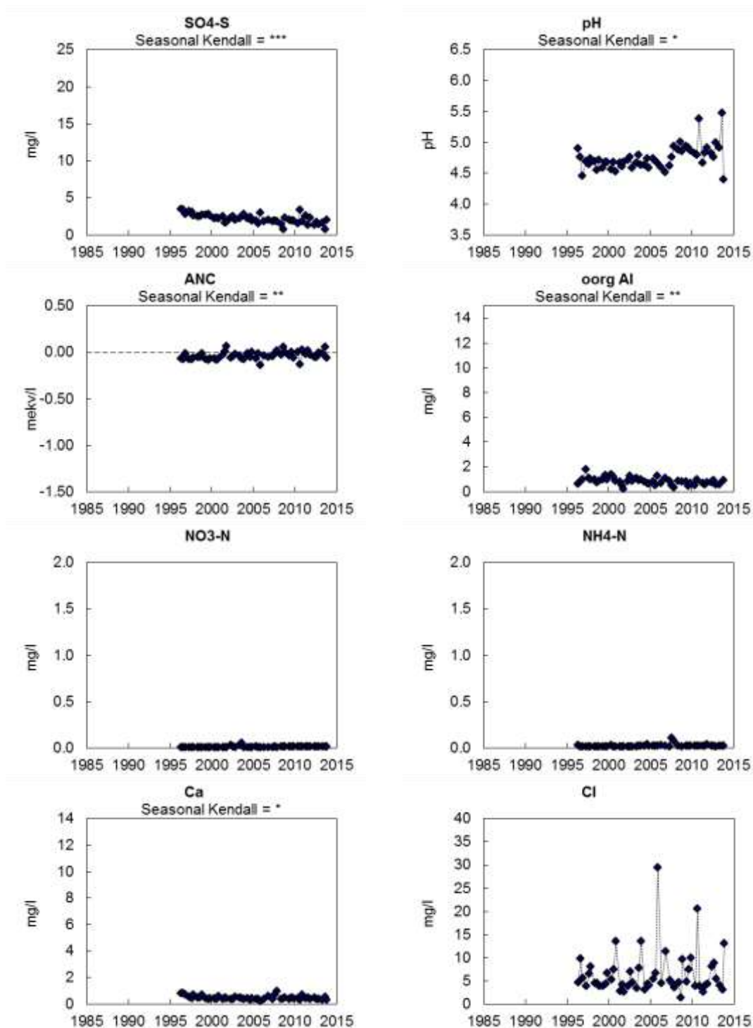
Figur B1:6. Markvattenkemi vid Komperskulla, K 11 . Sulfatsvavel (SO 4 -S); pH; markvattnets syraneutraliserande förmåga (ANC); oorganiskt aluminium (oorg Al); nitratkväve (NO 3 -N); ammoniumkväve (NH 4 -N), kalciumhalt (Ca 2+ ), samt klorid (Cl). Saknade värden innebär oftast att marken varit för torr. Trendanalys har genomförts med hjälp av Seasonal- Kendall metodik och signifikansnivåer anges, ovanför respektive diagram, i de fall där signifikanta trender påvisats.
