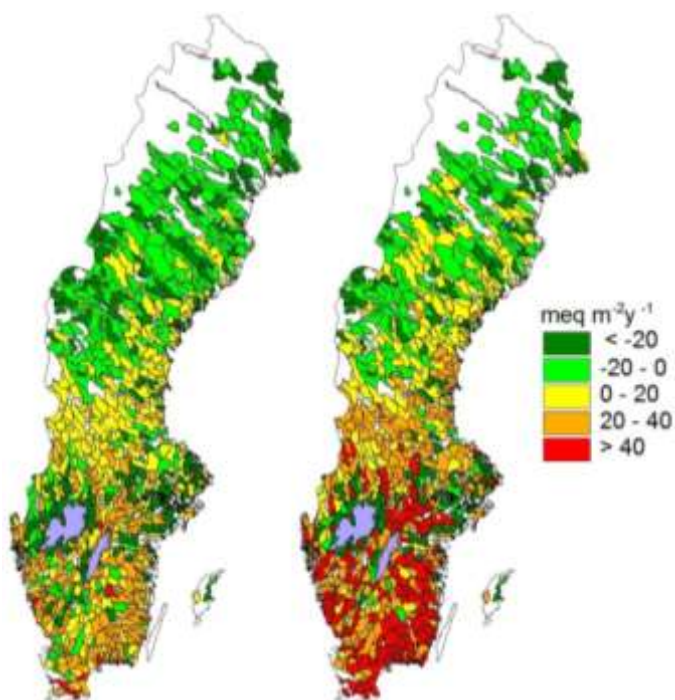
Figur 19. Överskridande av kritiskt baskatjonuttag i granskog vid stamuttag (a) och uttag av stam och grot (b).
