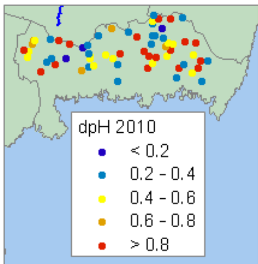
Figur 8. pH-förändring sedan förindustriell tid (dpH) i sjöar 2010, baserat på MAGIC-biblioteket. En sjö räknas som antropogent försurad om pH som årsmedian har sjunkit med minst 0,4 enheter sedan förindustriell tid (dpH > 0,4), vilket markeras med gula, orange och röda symbolerna på kartan. Analysen inkluderar kalkade försurade sjöar baserat på beräknad vattenkemi om man inte hade kalkat.
