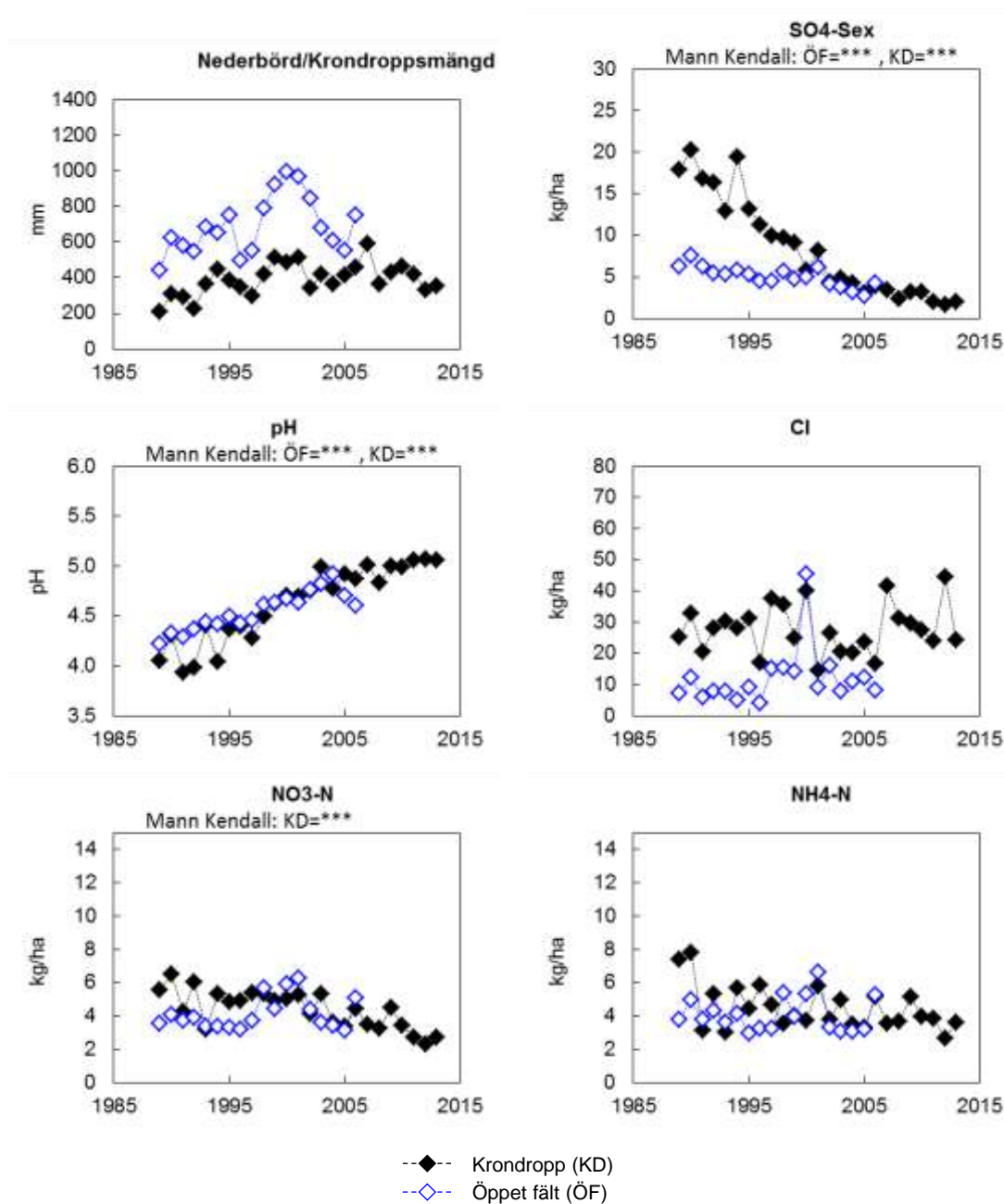
Figur B1:11. Årliga värden (hydrologiskt år) för depositionen via krondropp och över öppet fält vid Arkelstorp, L 05 . I figuren visas uppmätt nederbörd över öppet fält samt krondroppsmängder, uttryckt som mm. Deposition sedan mätningarna påbörjades redovisas för ett urval av ämnen: sulfatsvavel utan havssaltsbidrag (SO 4 -S ex), pH, kloridjoner (Cl), nitratkväve (NO 3 -N) och ammoniumkväve (NH 4 -N). ÖF, öppet fält; KD, krondropp. Trendanalys har genomförts med hjälp av Mann-Kendall- analys och signifikansnivåer anges, ovanför respektive diagram, i de fall där signifikanta trender påvisats.
