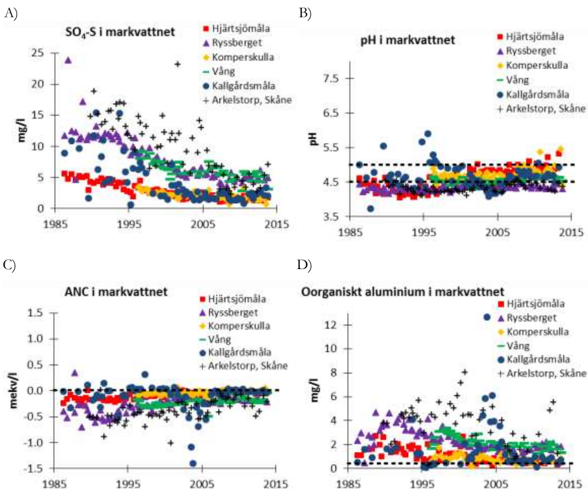
Figur 6. Halterna av A) sulfatsvavel (SO 4 -S), B) pH, C) syraneutraliserande förmåga (ANC) och D) halten oorganiskt aluminium (oorg-Al) i markvattnet på 50 cm djup vid olika platser i Blekinge län, samt vid Arkelstorp i Skåne, uppmätt inom Krondropps nätet. Följande förändringar är statistiskt säkerställda: SO 4 -S har minskat signifikant vid samtliga 6 ytor; pH och ANC har ökat vid samtliga ytor utom vid Kallgårdsmåla. Ooorg-Al har minskat vid samtliga ytor, utom vid Kallgårdsmåla och Arkelstorp. Streckade linjer anger försurningsgränser för pH, ANC och Ooorg-Al.
