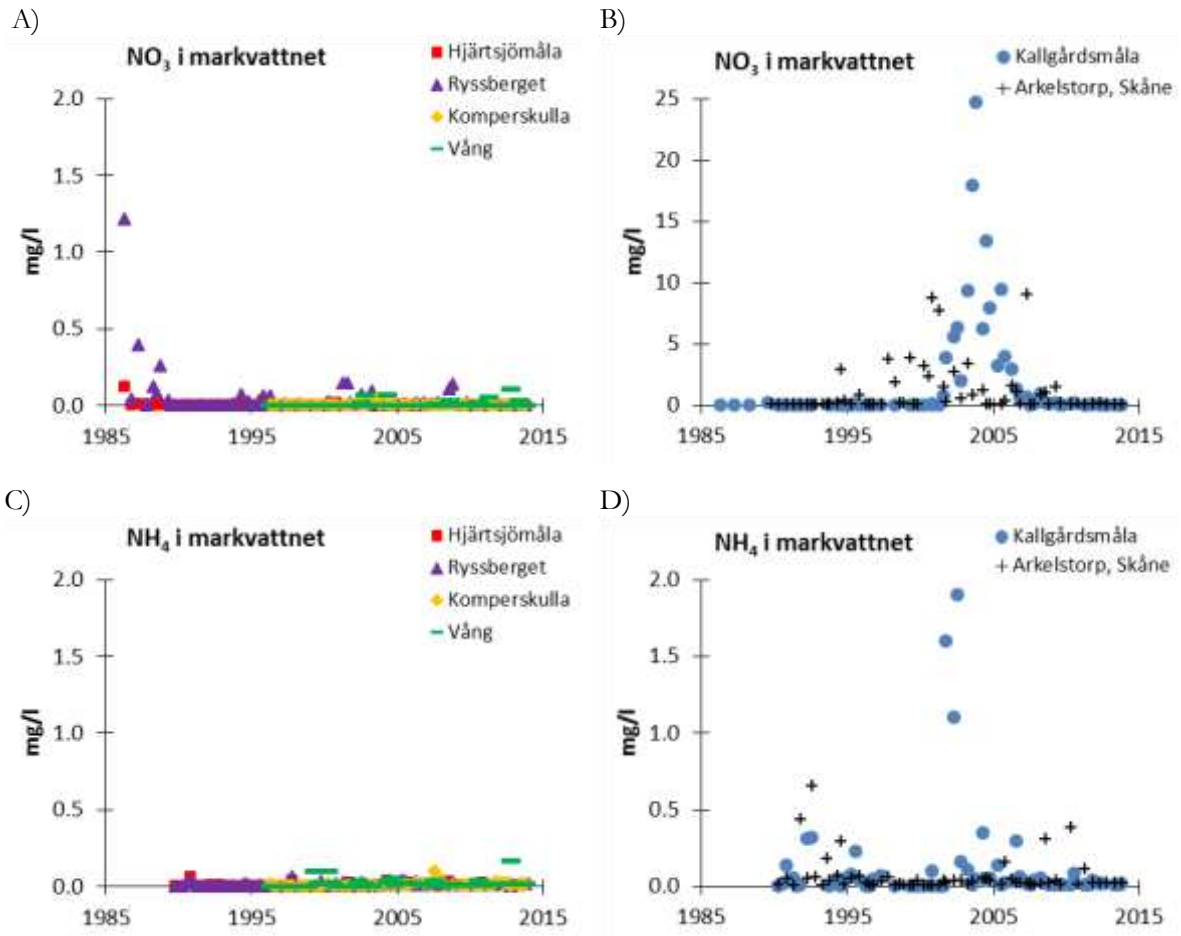
Figur 11. Halterna i markvattnet på 50 cm djup vid olika platser i Blekinge län av A - B) nitratkväve ( \text{NO}_3\text{-N} ) i markvattnet, samt C-D) halterna av ammoniumkväve ( \text{NH}_4\text{-N} ) i markvattnet. Vid Kallgårdsmåla avverkades skogen år 2000, och Kallgårdsmåla visas därför i ett separat diagram med annan skala på y-axeln. Även Arkelstorp i Skåne visas tillsammans med Kallgårdsmåla, eftersom denna yta i nordöstra Skåne har förhållandevis höga nitratvärden. Inga förändringar är statistiskt säkerställda.
