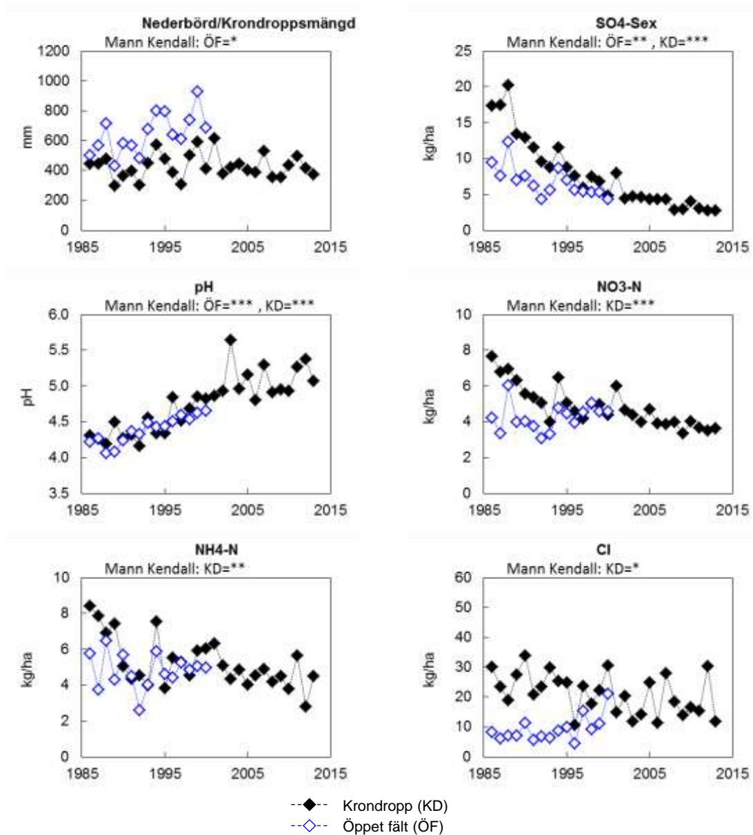
Figur B1:3. Årliga värden (hydrologiskt år) för depositionen via krondropp och över öppet fält vid Ryssberget, K 07 . I figuren visas uppmätt nederbörd över öppet fält samt krondroppsmängder, uttryckt som mm. Deposition redovisas sedan mätningarna påbörjades för ett urval av ämnen: sulfatsvavel utan havssaltsbidrag (SO 4 -S ex); pH; nitratkväve (NO 3 -N); ammoniumkväve (NH 4 -N); kloridjoner (Cl - ). ÖF, öppet fält; KD, krondropp. Trendanalys har genomförts med hjälp av Mann-Kendall metodik och signifikansnivåer anges, ovanför respektive diagram, i de fall där signifikanta trender påvisats.
