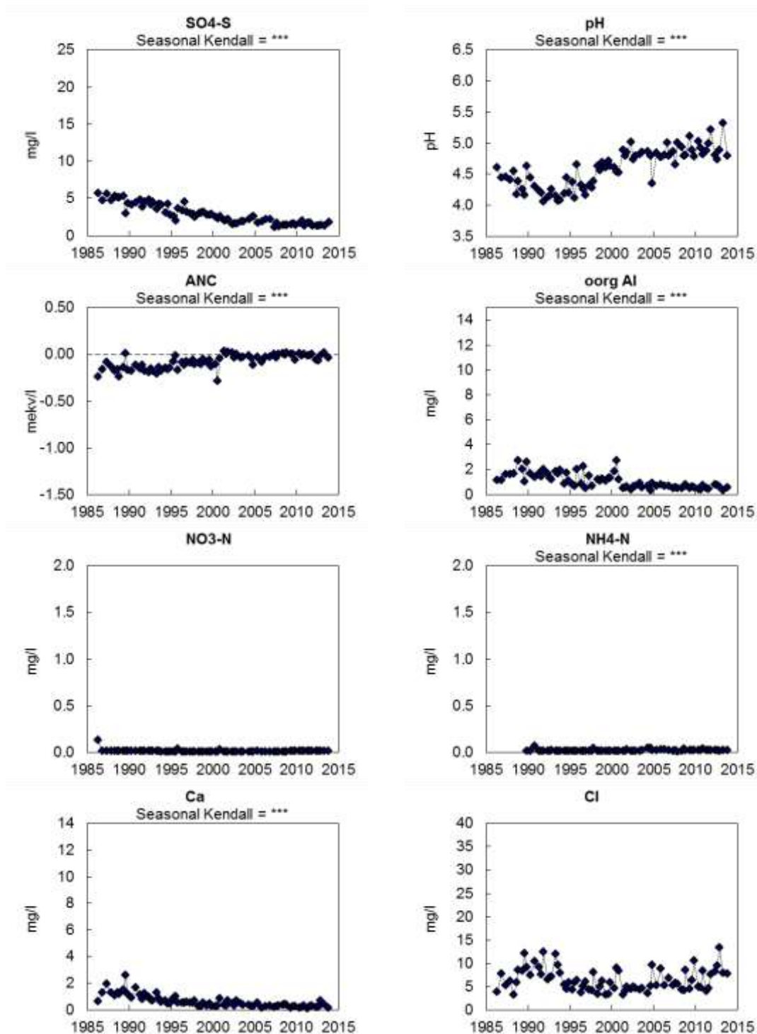
Figur B1:2. Markvattenkemi vid Hjärtsjömåla, K 03 . Sulfatsvavel (SO 4 -S); pH; markvattnets syraneutraliserande förmåga (ANC); oorganiskt aluminium (oorg Al); nitratkväve (NO 3 -N); ammoniumkväve (NH 4 -N); kalciumhalt (Ca 2+ ); kloridhalt (Cl). Saknade värden innebär oftast att marken varit för torr. Trendanalys har genomförts med hjälp av Seasonal-Kendall metodik och signifikansnivåer anges, ovanför respektive diagram, i de fall där signifikanta trender påvisats.
