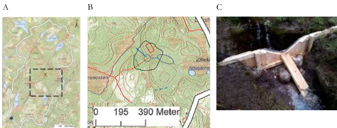
Figur 17. A, Avrinningsområdet Sägebäcken. Avrinningsområdet avgränsas av den breda vita linjen. ● Befintliga ytvattenmätningar i Sägebäcken som avvattnar hela avrinningsområdet (finansierat av Länsstyrelsen i Västra Götaland). B, En uppförstoring (från figur A) av ett mindre delavrinningsområde i anslutning till krondroppsytan. En svart oregelbunden linje indikerar avgränsningen för delavrinningsområdet. En tjockare blå linje visar bäcken där provtagningen av bäckvatten sker. En tjock röd rektangel visar krondroppsytan. Blå cirklar indikerar sankmarker. C, Ett foto av den nyanlagda dammen (2014-04-10).
