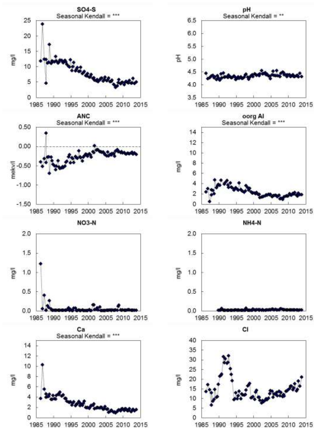
Figur B1:4. Markvattenkemi vid Ryssberget, K 07 . Sulfatsvavel (SO4-S); pH; markvattnets syraneutraliserande förmåga (ANC); oorganiskt aluminium (oorg Al); nitratkväve (NO3-N); ammoniumkväve (NH4-N), kalciumhalt (Ca 2+ ), samt klorid (Cl). Saknade värden innebär oftast att marken varit för torr. Trendanalys har genomförts med hjälp av Seasonal- Kendall metodik och signifikansnivåer anges, ovanför respektive diagram, i de fall där signifikanta trender påvisats.
