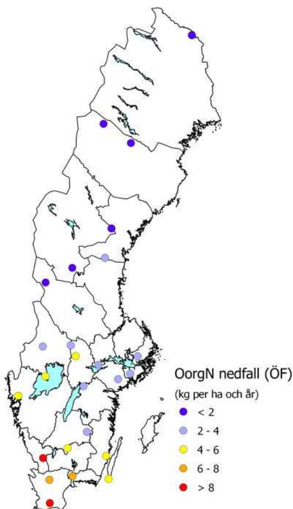
Figur 9. Nedfallet av oorganiskt kväve (oorgN) med nederbörden till öppet fält vid olika platser inom Krondroppsnetet under det hydrologiska året 2012/13.
