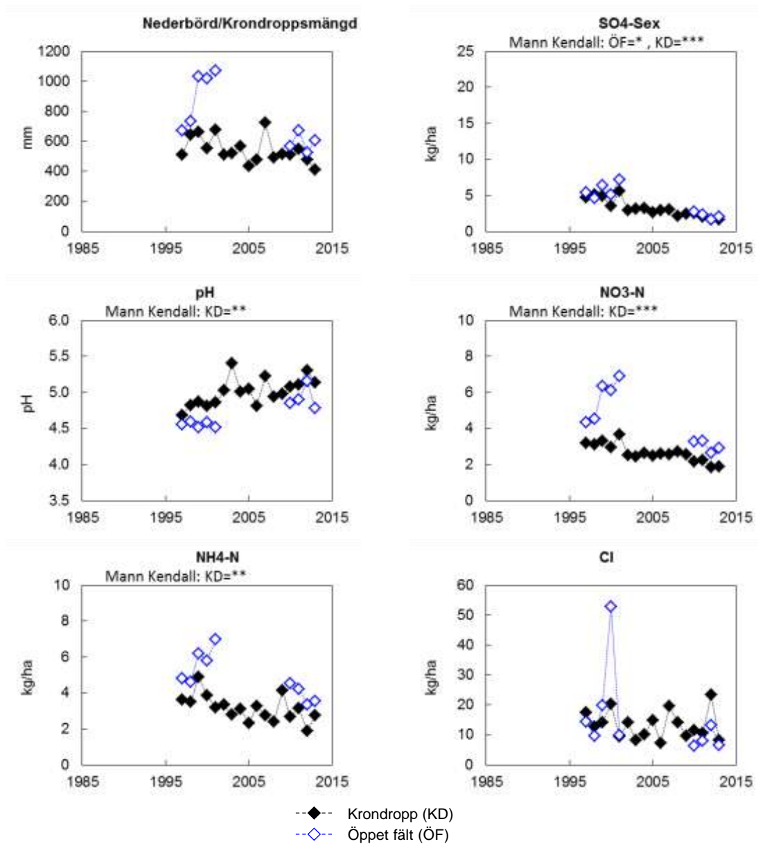
Figur B1:5. Årliga värden (hydrologiskt år) för depositionen via krondropp och över öppet fält vid Komperskulla, K 11 . I figuren visas uppmätt nederbörd över öppet fält samt krondropps- mängder, uttryckt som mm. Deposition redovisas sedan mätningarna påbörjades för ett urval av ämnen: sulfatsvavel utan havssaltsbidrag (SO 4 -S ex); pH; nitratkväve (NO 3 -N); ammoniumkväve (NH 4 -N); kloridjoner (Cl). ÖF, öppet fält; KD, krondropp. Trendanalys har genomförts med hjälp av Mann-Kendall metodik och signifikansnivåer anges, ovanför respektive diagram, i de fall där signifikanta trender påvisats.
