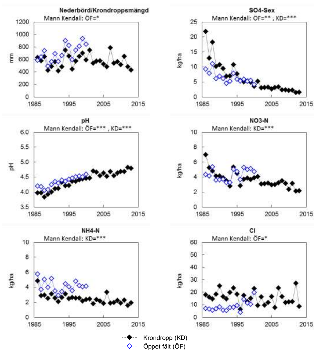
Figur B1:1. Årliga värden (hydrologiskt år) för depositionen via krondropp och över öppet fält vid Hjärtsjömåla, K 03. I figuren visas uppmätt nederbörd över öppet fält samt krondroppsmängder, uttryckt som mm. Deposition redovisas sedan mätningarna påbörjades för ett urval av ämnen: sulfatsvavel utan havssaltsbidrag (SO4-S ex); pH; nitratkväve (NO3-N); ammoniumkväve (NH4-N); kloridjoner (Cl-). ÖF, öppet fält; KD, krondropp. Trendanalys har genomförts med hjälp av Mann- Kendall metodik och signifikansnivåer anges, ovanför respektive diagram, i de fall där signifikanta trender påvisats.
