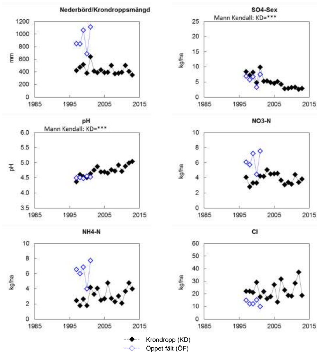
Figur B1:7. Årliga värden (hydrologiskt år) för depositionen via krondropp och över öppet fält vid Vång, K 13 . I figuren visas uppmätt nederbörd över öppet fält samt krondroppsmängder, uttryckt som mm. Deposition redovisas sedan mätningarna påbörjades för ett urval av ämnen: sulfatsvavel utan havssaltsbidrag (SO 4 -S ex); pH; nitratkväve (NO 3 -N); ammoniumkväve (NH 4 -N); kloridjoner (Cl). ÖF, öppet fält; KD, krondropp. Trendanalys har genomförts med hjälp av Mann-Kendall metodik och signifikansnivåer anges, ovanför respektive diagram, i de fall där signifikanta trender påvisats.
