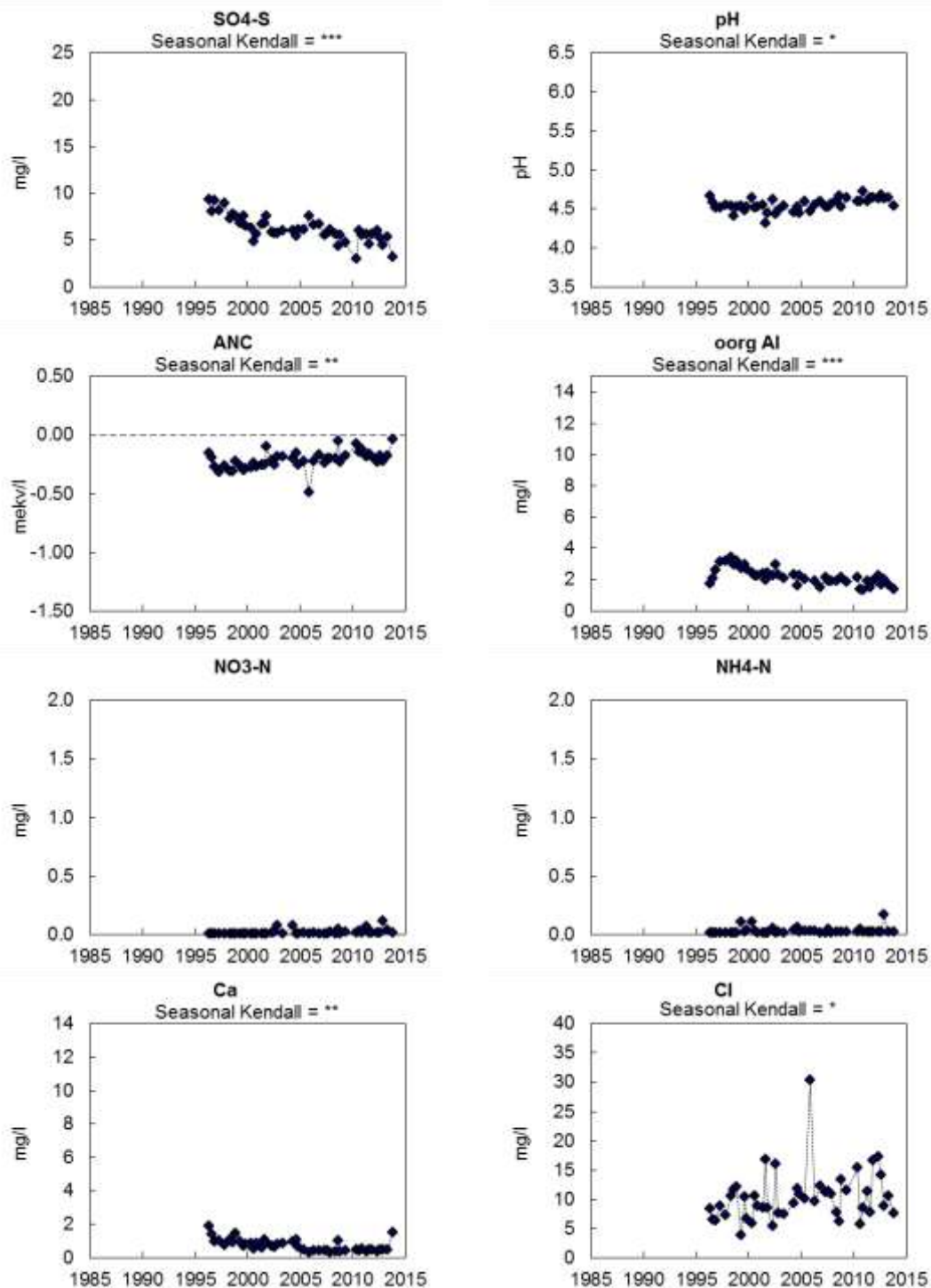
Figur B1:8. Markvattenkemi vid Vång, K 13. Sulfatsvavel (SO4-S); pH; markvattnets syraneutraliserande förmåga (ANC); oorganiskt aluminium (oorg Al); nitratkväve (NO3-N); ammoniumkväve (NH4-N); kalciumhalt (Ca 2+ ), samt klorid (Cl). Saknade värden innebär oftast att marken varit för torr. Trendanalys har genomförts med hjälp av Seasonal- Kendall metodik och signifikansnivåer anges, ovanför respektive diagram, i de fall där signifikanta trender påvisats.
